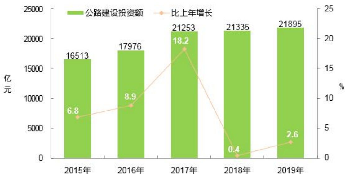
图9 2015—2019年公路建设投资额及增长速度
